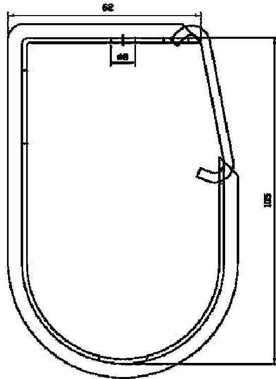
Seitenansicht
