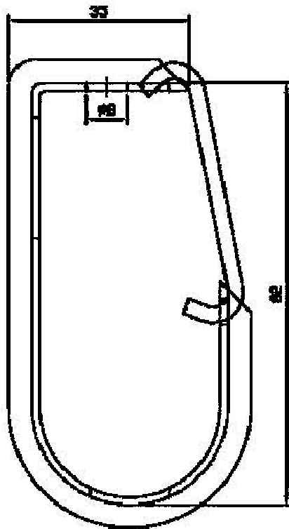
Seitenansicht
